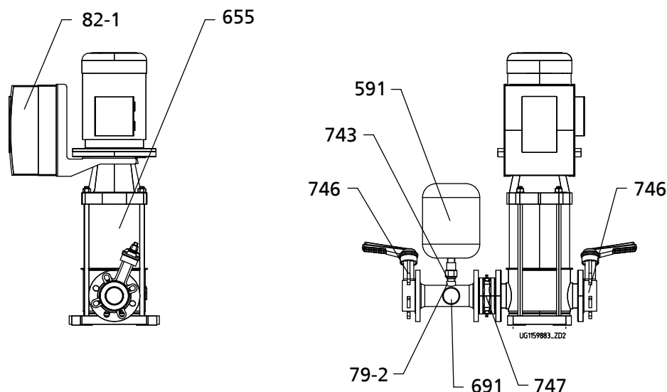
Рисунок 16: Общий вид Hya-Solo DV с Movitec 32, 45, 65, 90
