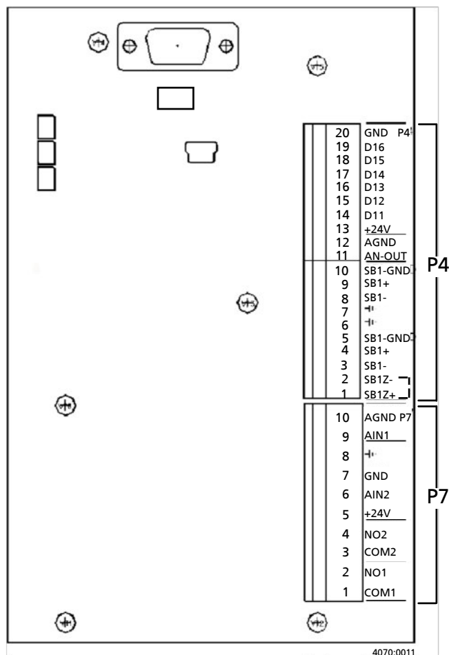
Рисунок 7: Клеммы управления вводов/выводов
