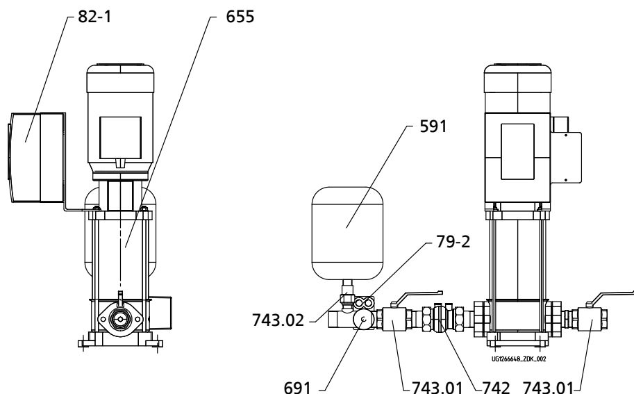
Рисунок 15: Общий вид Нya-Solo DV с Movitec 2, 4, 6, 10, 18
