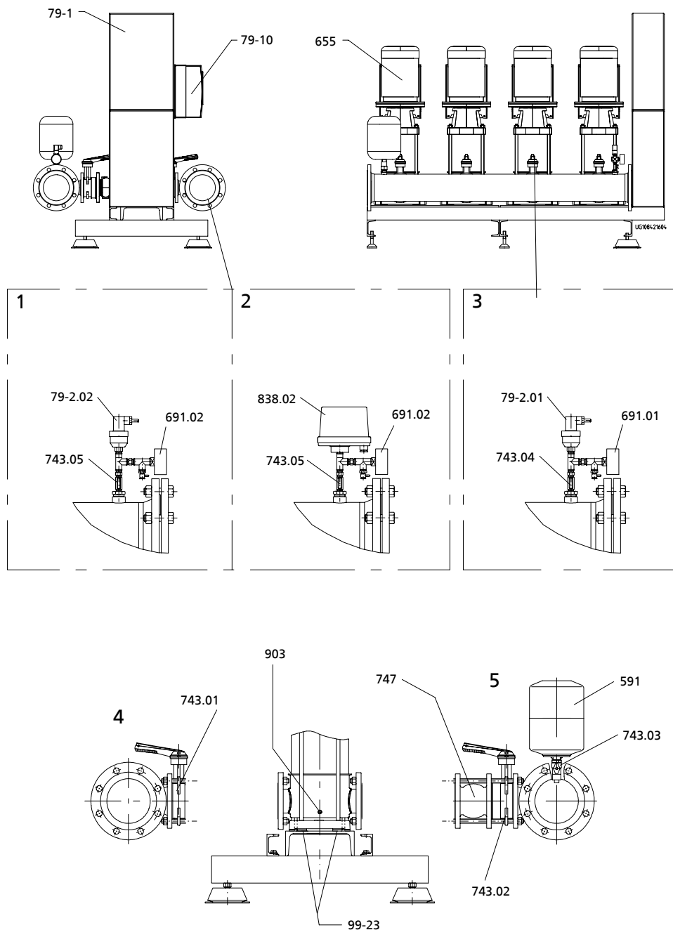
Рисунок 14: Запасные части для Hyamat VP с Movitec 32, 45, 65, 90
