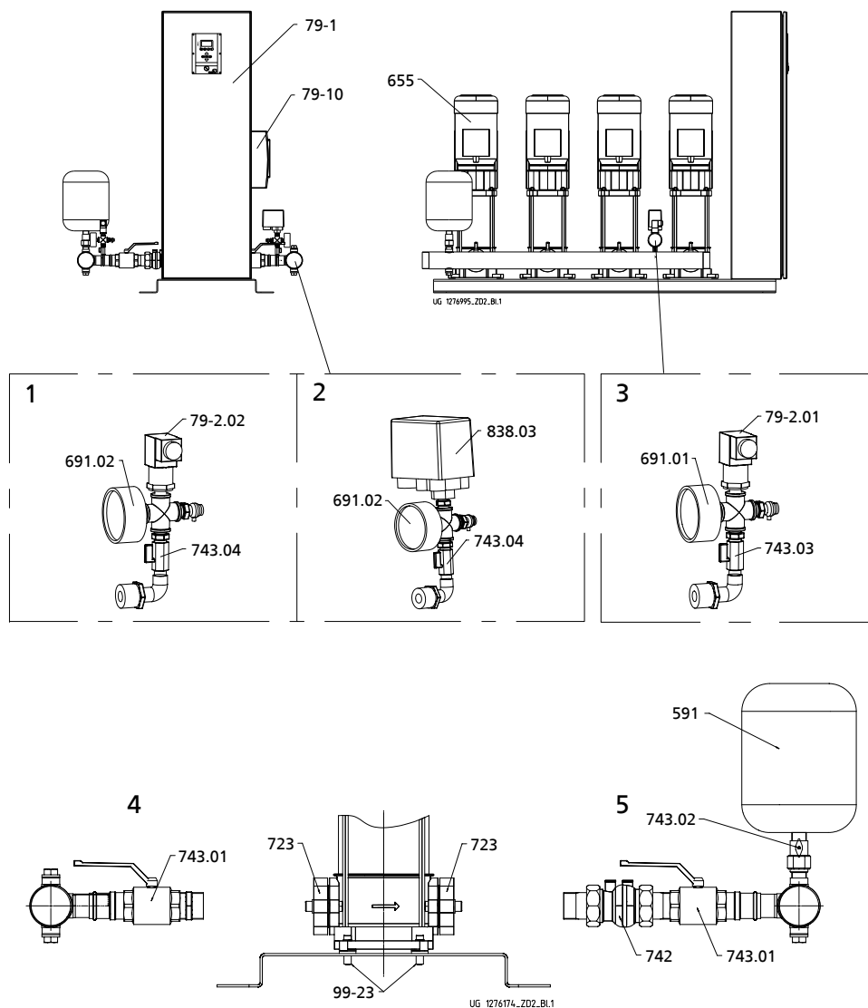
Рисунок 13: Запасные части для Hyamat VP с Movitec 2, 4, 6, 10, 18
