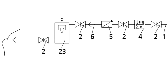
Рисунок 16: Технологическая схема, опосредованное подключение
