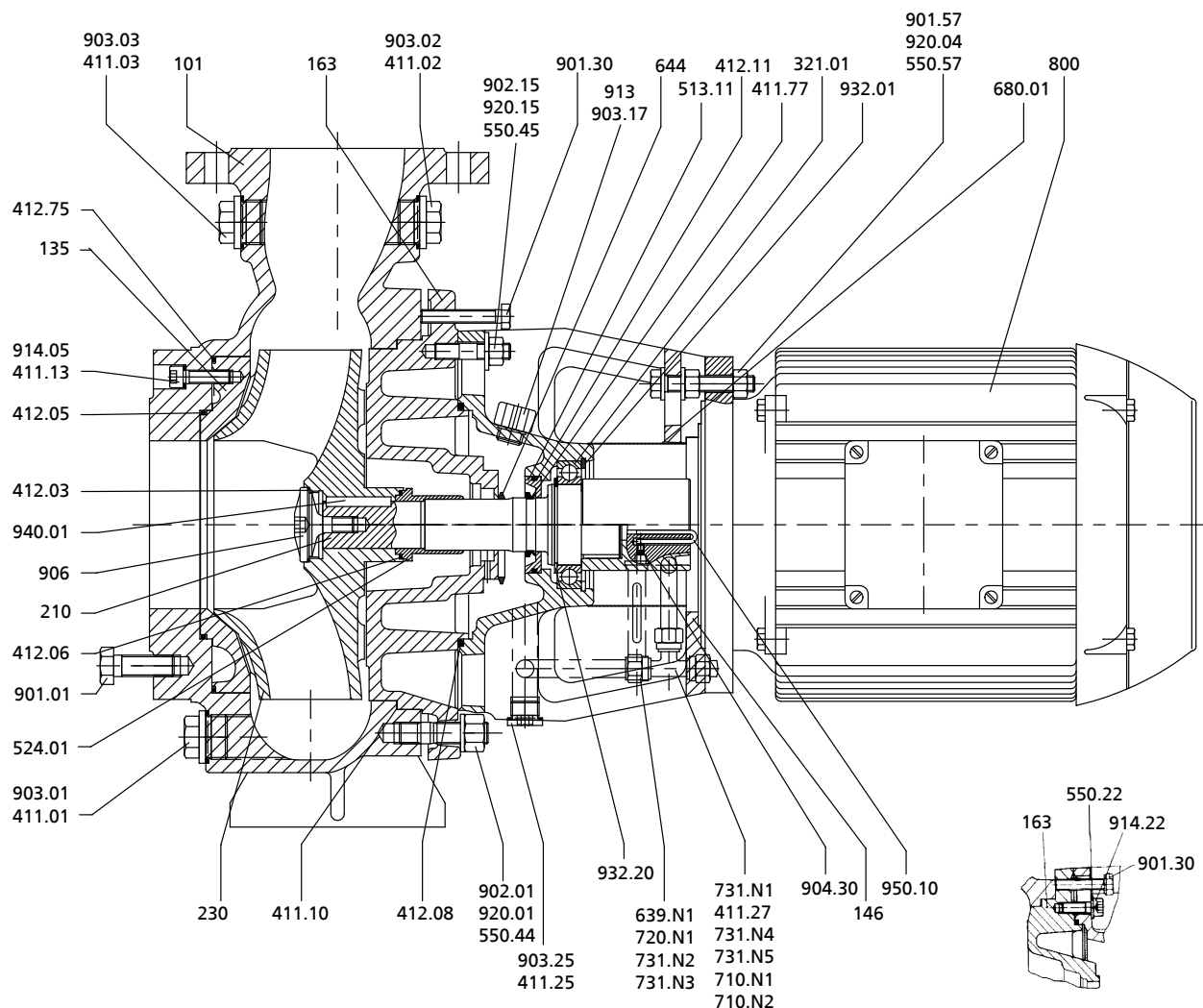
Рисунок 8: Общий чертеж с перечнем деталей KWP-Bloc модель GN, GC2
