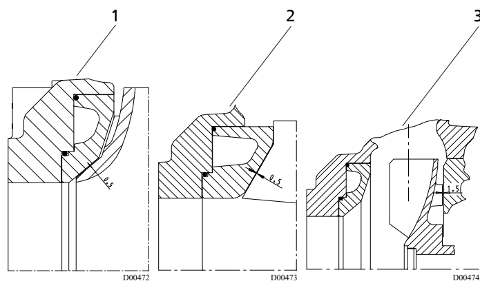
Рисунок 3: Зазоры
